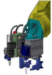
04 Robot gripper
