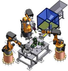
01 Prüfstation
